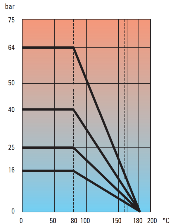
Diagramme pression-température (PTFE)
